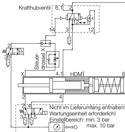
HDM = Hochdruckmessanschluss
