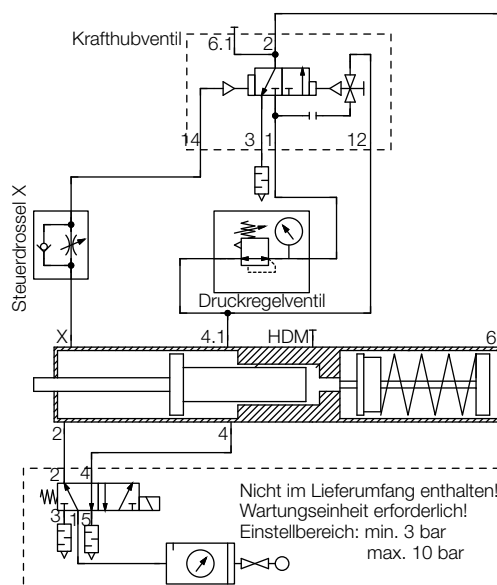
HDM = Hochdruckmessanschluss
